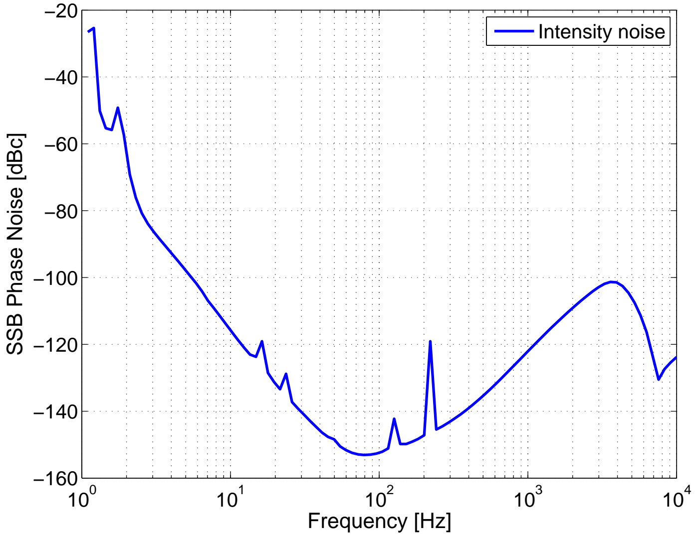
f1 SSB Phase Noise Requirement (Safety Factor 20 dBc)
