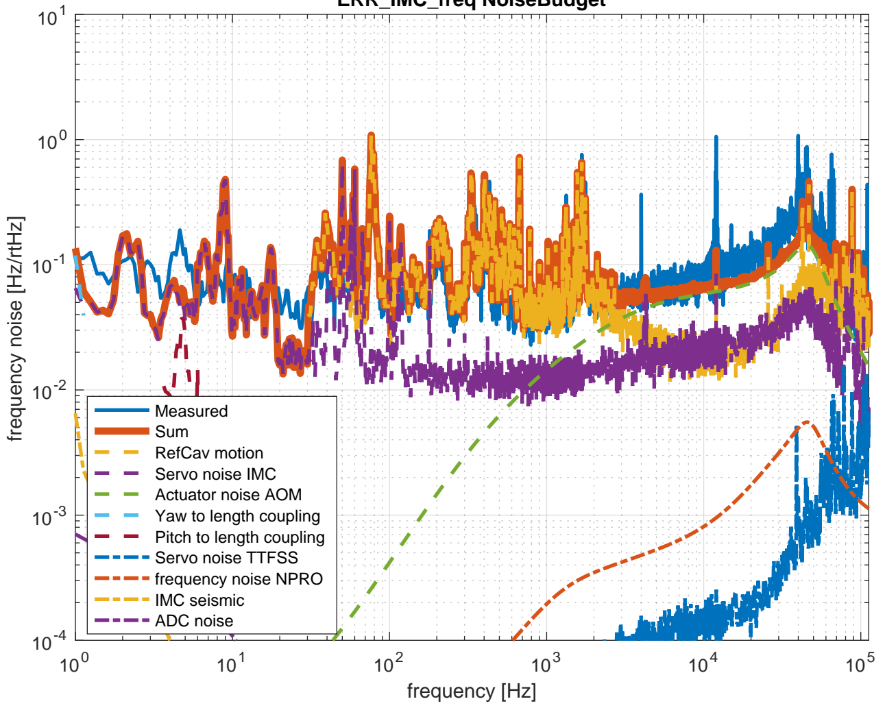
ERR_IMC_freq NoiseBudget
