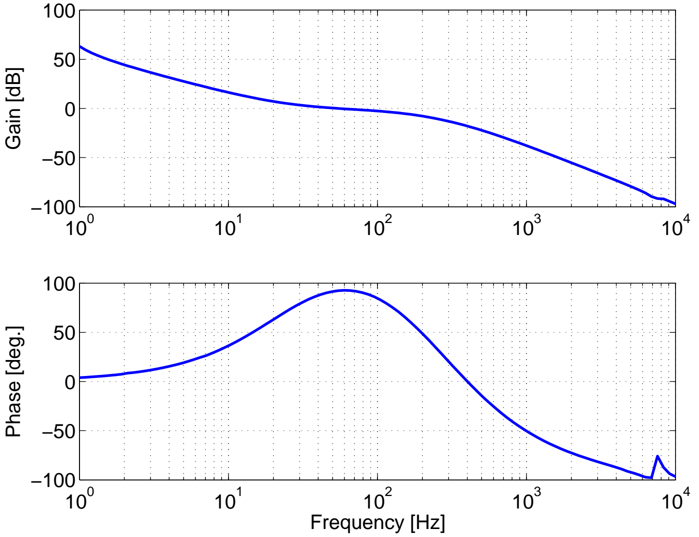
MICH Open Loop Gain
