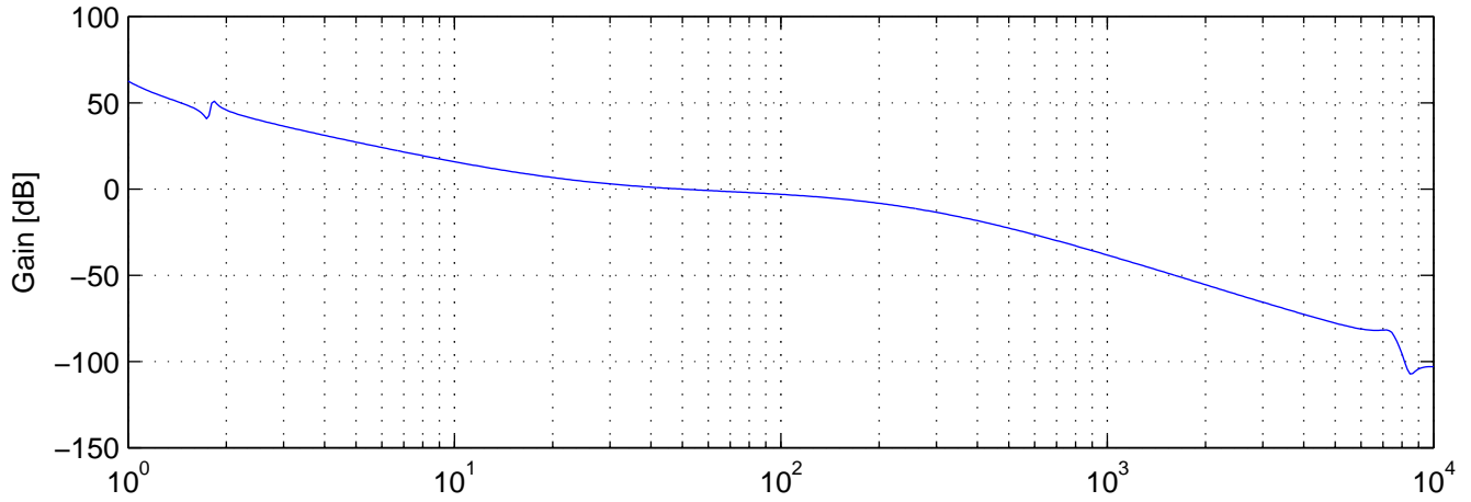
MICH Open Loop Gain
