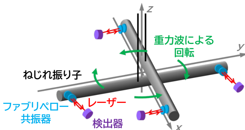
図1: TOBA の構成。
