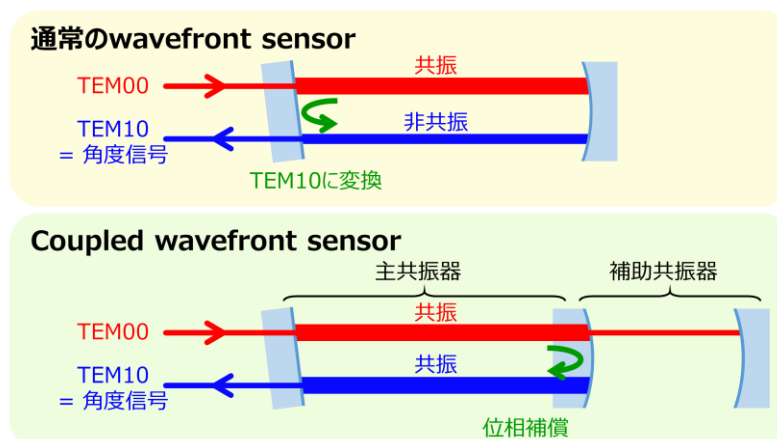
図: 通常の wavefront sensor の構成(上)と Coupled wavefront sensor の構成(下)。
