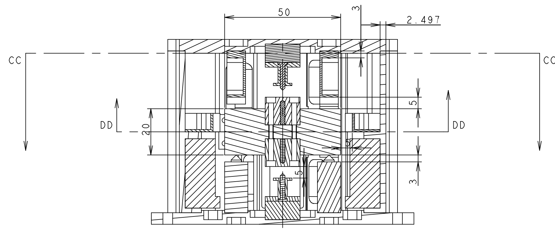
断面 AA-AA
