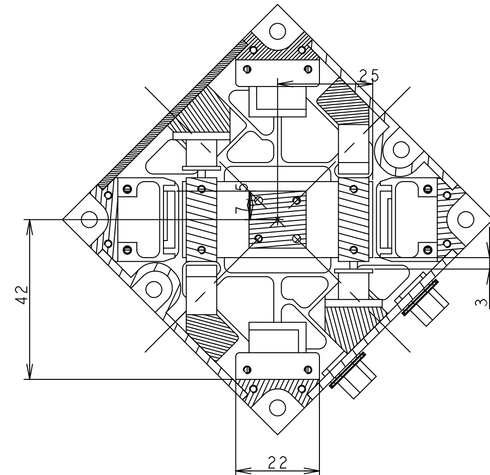
断面 CC-CC
