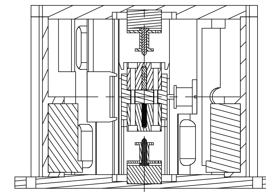
断面 BB-BB
