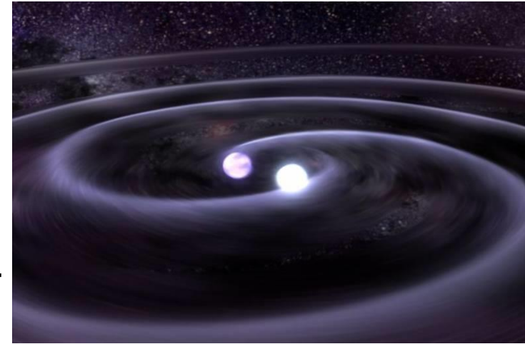
連星ブラックホール
