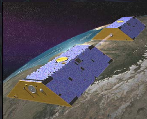
GRACE (NASA, 2002-)
